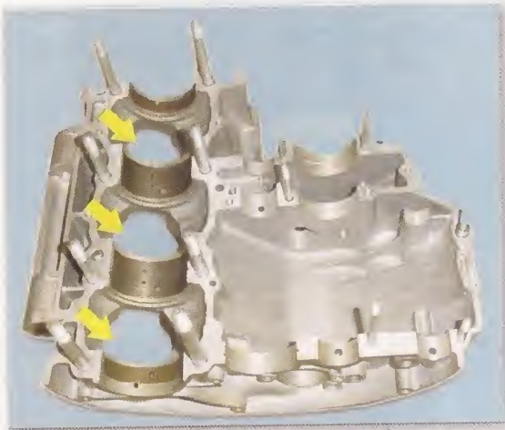
Carter de motor policilindrico
